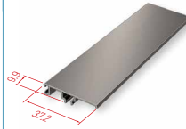
F85-1K51 Bitiş kapak profili Base cover
