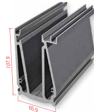
F85-460 Taşıyıcı baza profili Wedge profile
