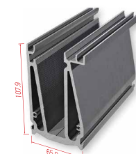
F85-460 Taşıyıcı baza profili Wedge profile
