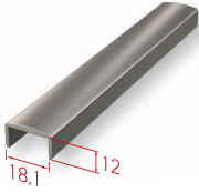
17.52mm için U küpeşte Handrail 17.52mm
