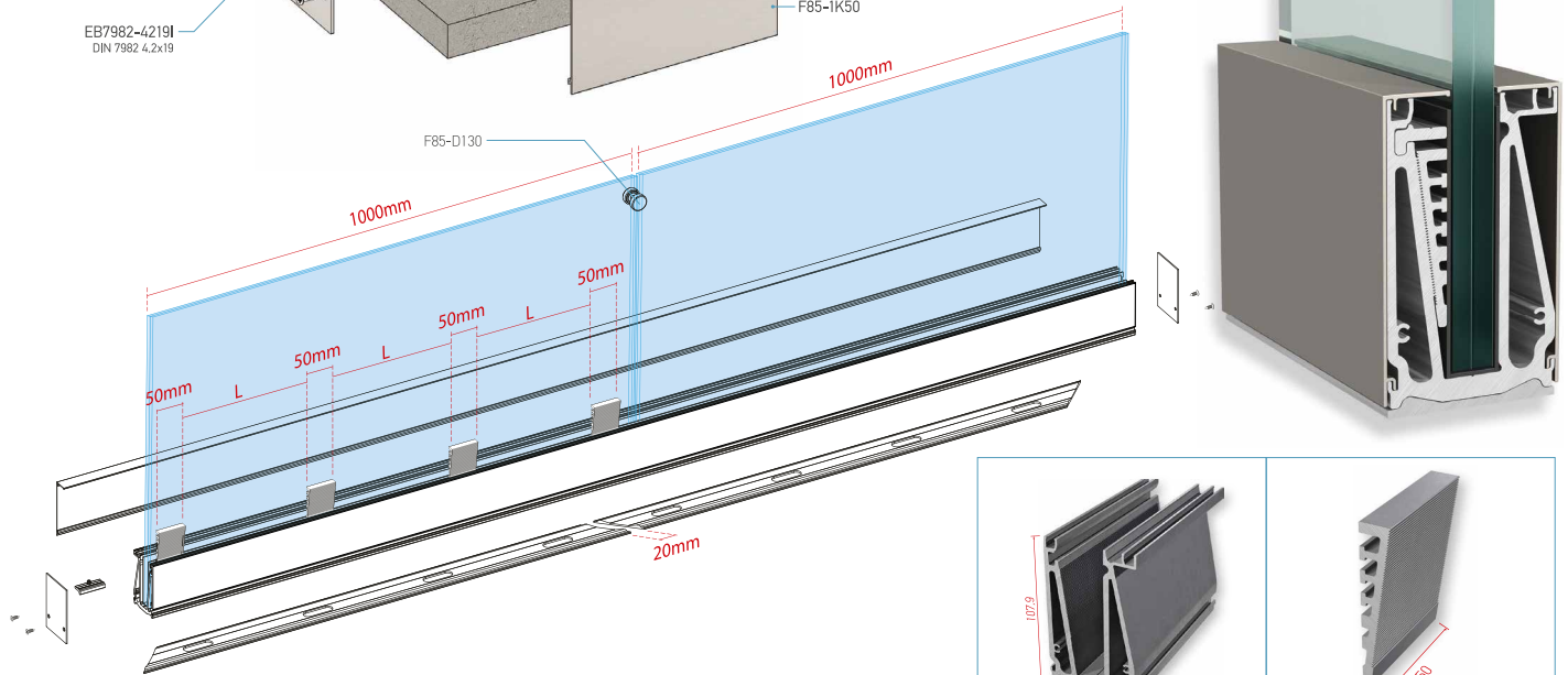
F85-460 Taşıyıcı baza profili Wedge profile
